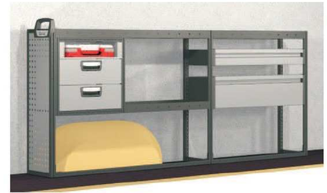
Best.Nr. Breite Höhe Tiefe Gewicht 203424112 2025 918 324 41
