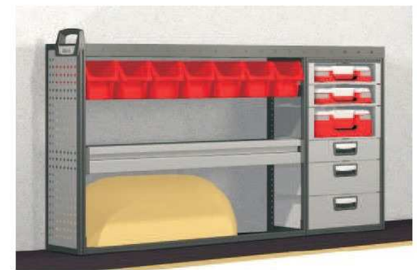
Best.Nr. Breite Höhe Tiefe Gewicht 203424107 1674 918 324 47
